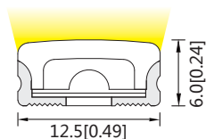
截面示意图：
