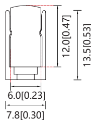
安装铝槽 型号：ASY-NSF0612-A1(A3)NNXXXX-MT
