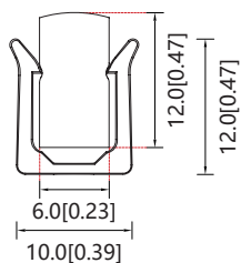
塑胶安装槽 型号：ASY-NSF0612-P1NNXXXX-MT
