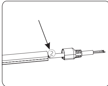
②. 先在堵头内部打防水胶，再推入灯带；
