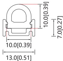
铝槽 / 铝卡 型号：ASY-NDR1010-A1(A3)NNXXXX-MT
